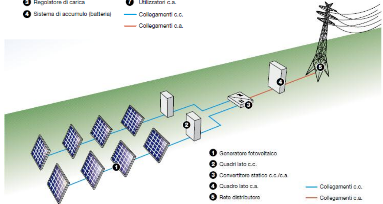
Impianti "grid connected"
